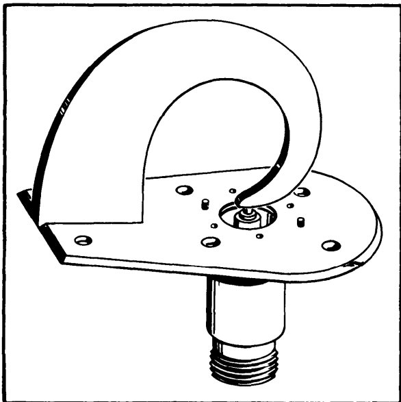
Figure 4-12. Scimitar Antenna.
